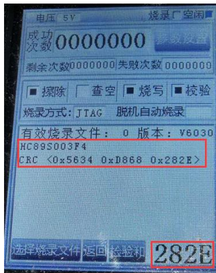
图 3.2-5 HC-PM51-V6 显示屏确认芯片型号及 CRC，LED 亮绿灯
