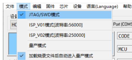
图 4-1 菜单栏切换至 JTAG/SWD 模式 (根据实际需要)
