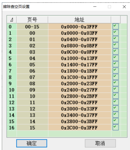
图 4.7-2 擦除查空页设置
