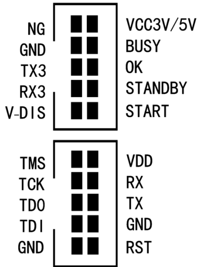
图 2-1 HC-PM51-V6 硬件引脚图
