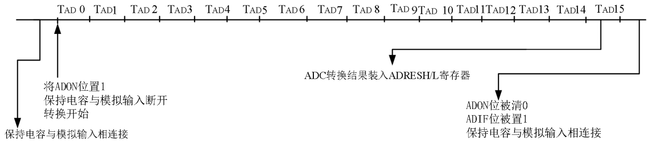
ADC转换时间(TAD)与工作频率关系表
