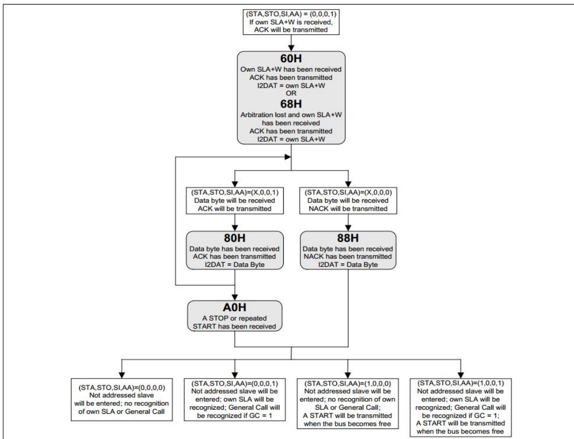
Figure 17- 12 从机接收模式流程与状态
