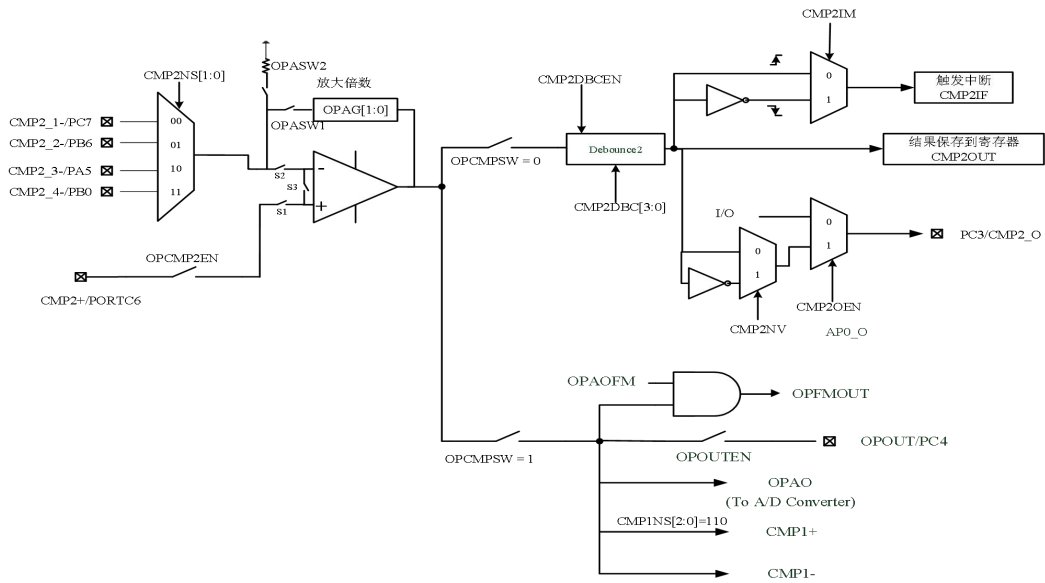
图11-1: CMP2和OP的功能框图
