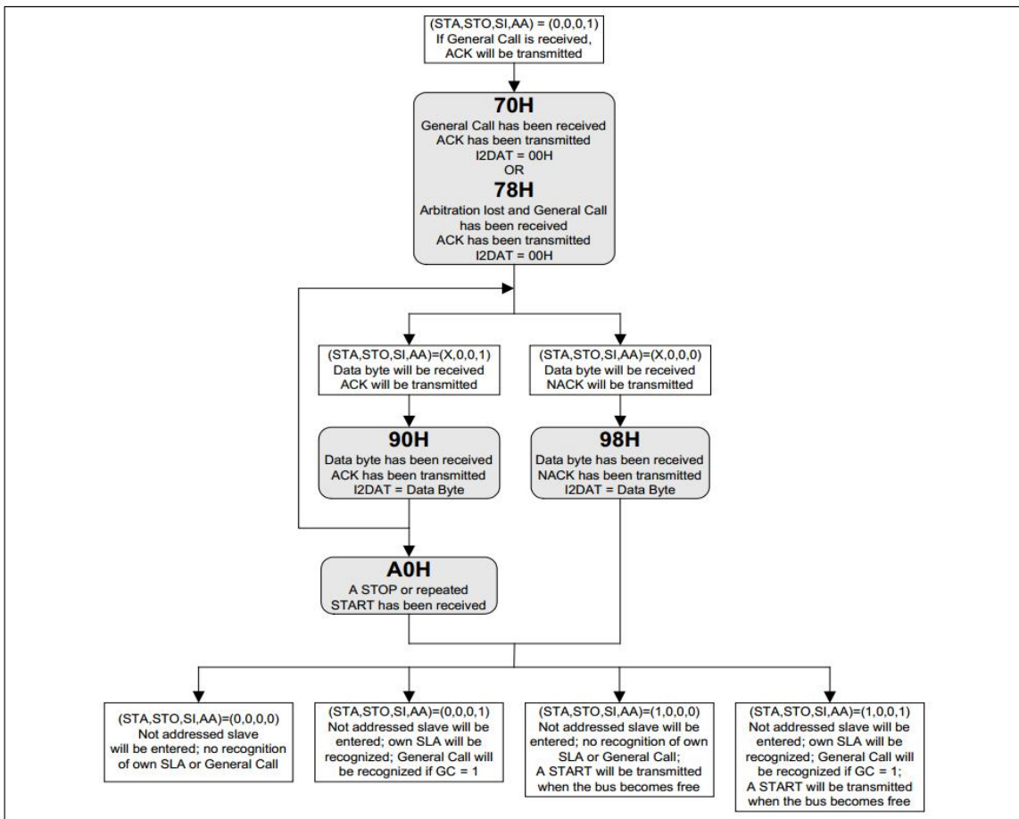
Figure 17- 13 广播呼叫模式流程与状态
