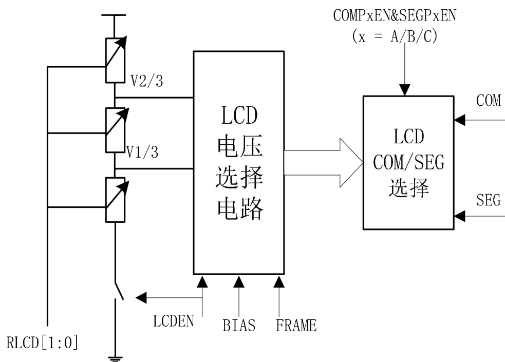
Figure 18-1 LCD 系统框图
