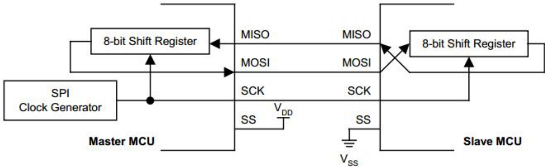
Figure 16- 2 全双工主从互联图
