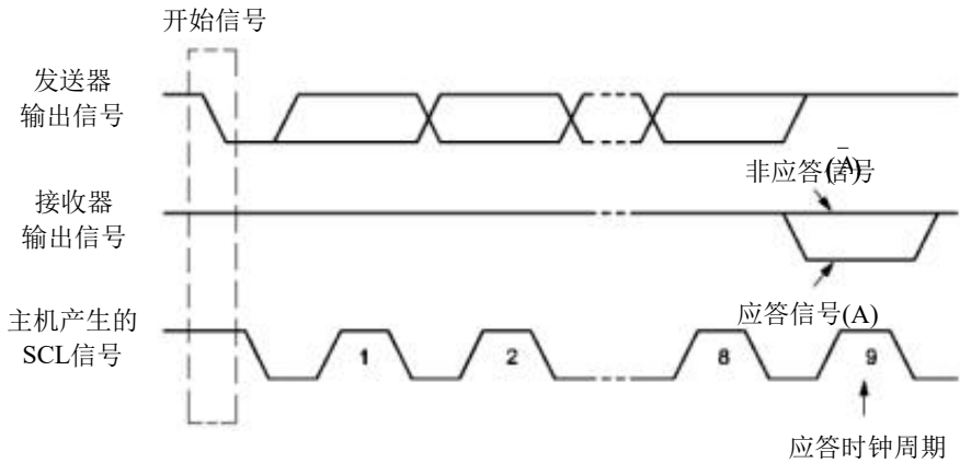
Figure 17-5 IIC 总线的应答信号
