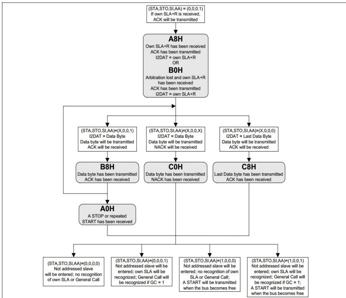
Figure 17- 11 从机发送模式流程与状态
