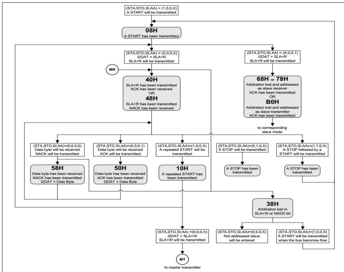
Figure 17-10 主机接收模式流程与状态
