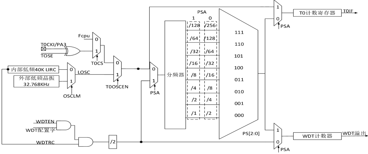
T0 控制寄存器 T0CON
