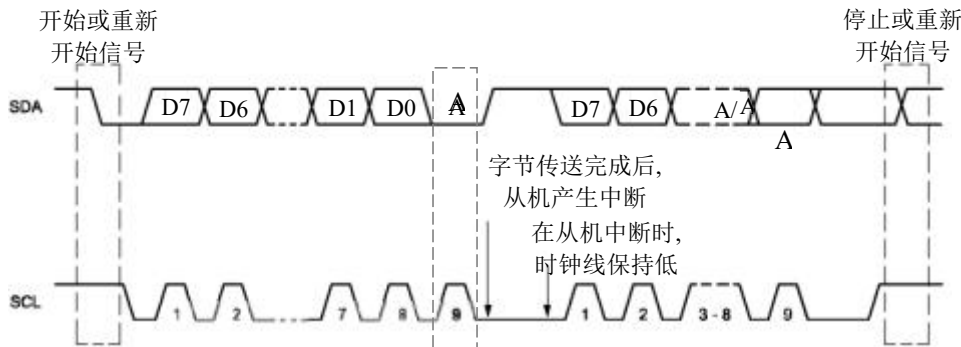
Figure 17-6 IIC 总线的数据传输格式
