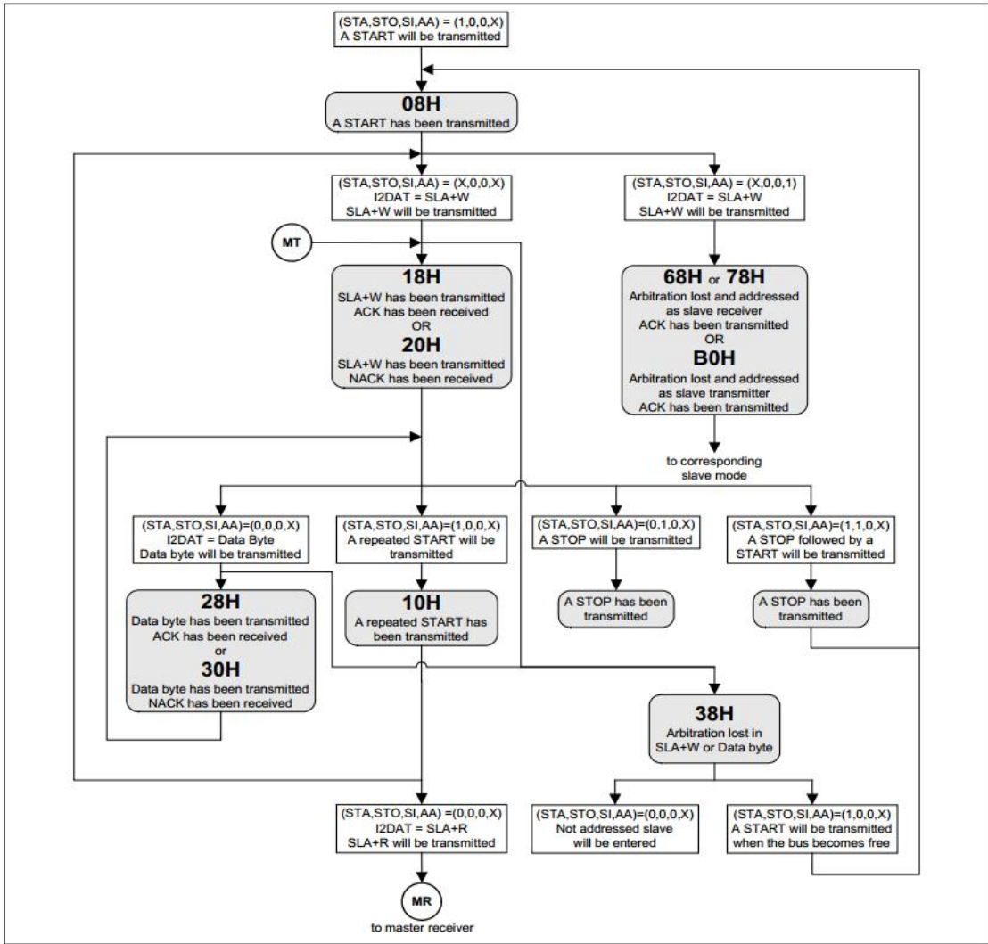
Figure 17-9 主机发送模式流程与状态
