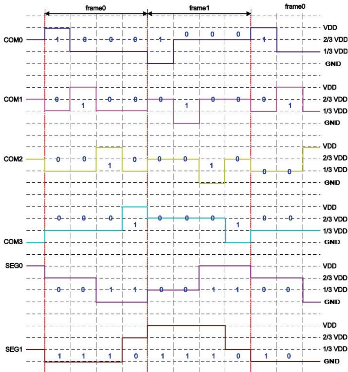
Figure 18-3 1/3bias LCD 波形图
