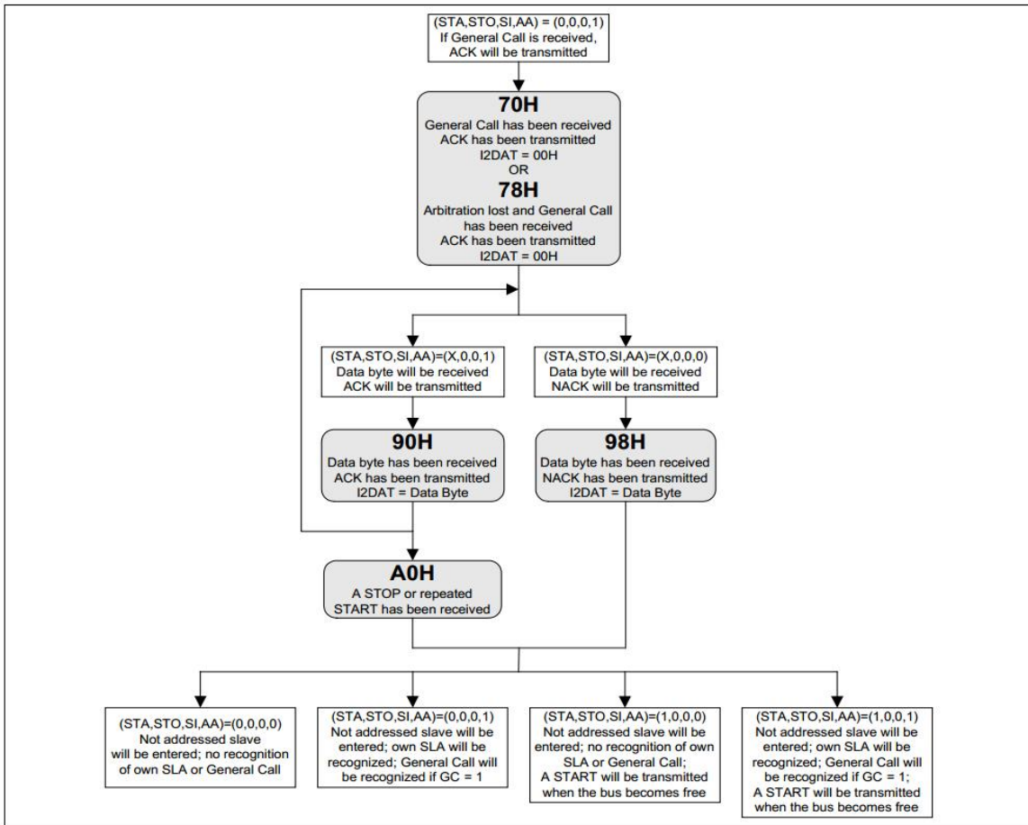
Figure 17-13 广播呼叫模式流程与状态
