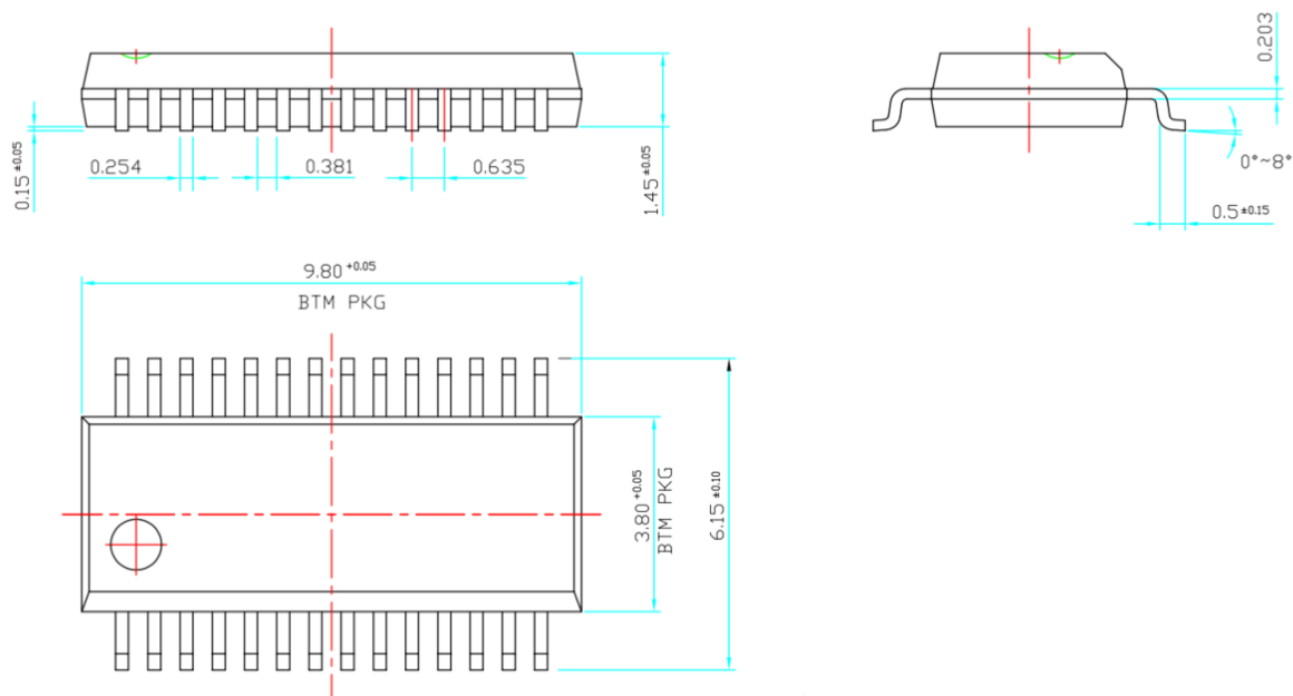
Figure 21-5 TSSOP20 封装尺寸
