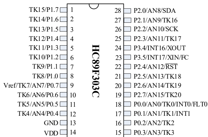
Figure 1-2 SOP28/SSOP28 引脚配置图
