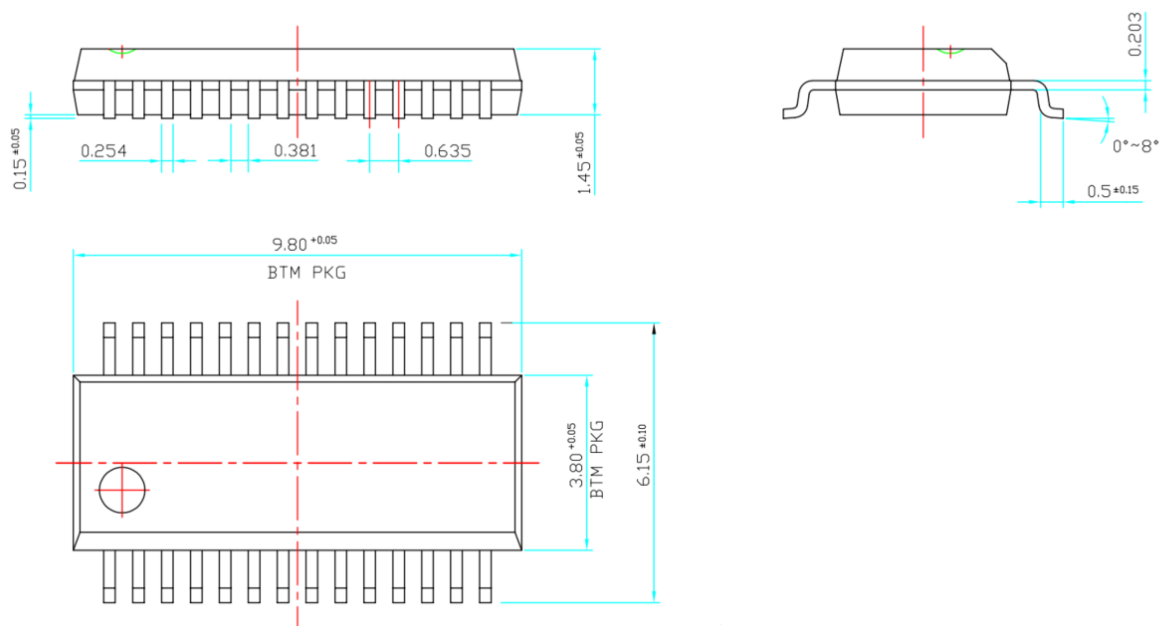
Figure 21-2 SSOP28 封装尺寸
