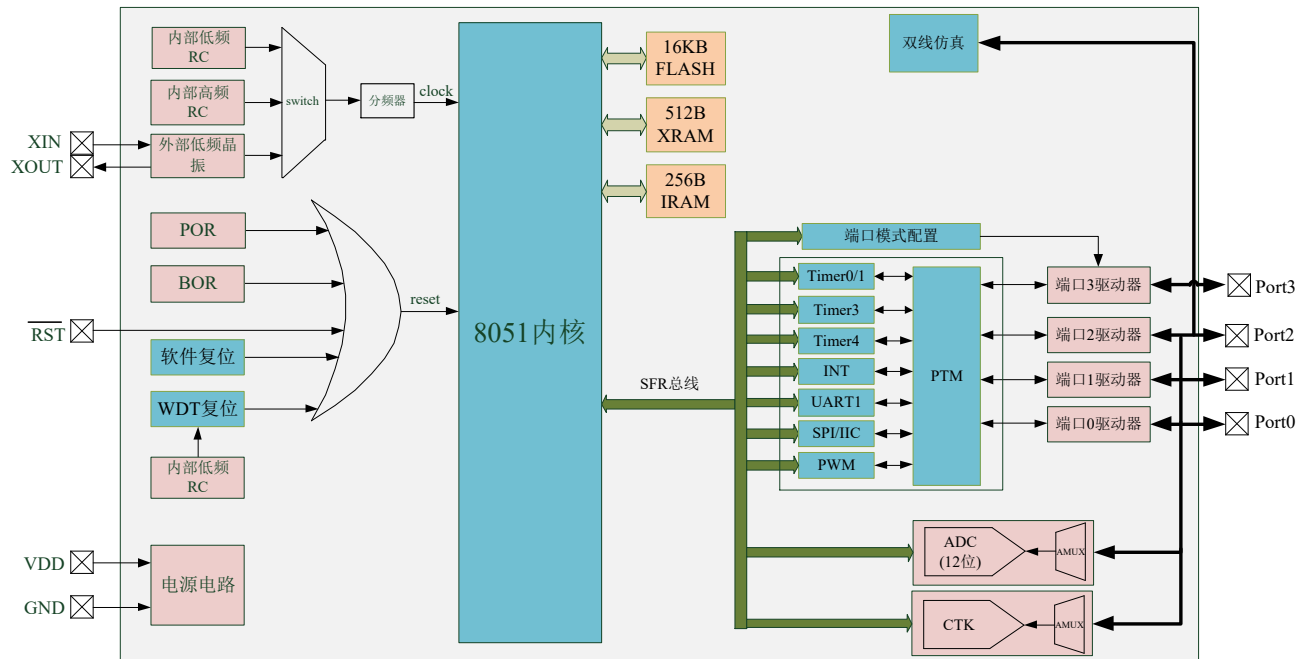
Figure 1-1 系统框图
