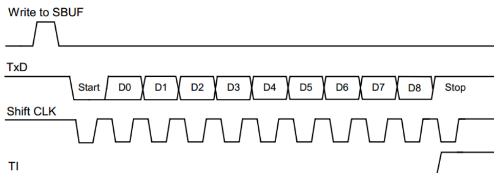
任何将 SBUF 作为目标寄存器的写操作都会启动发送，同时也将 TB8 载入到发送移位寄存器的第 9 位中。实际上发送是从 16 分频计数器中的下一次跳变之后的系统时钟开始的，因此位时间与 16 分频计数器是同步的，与对 SBUF 的写操作不同步。起始位首先在 TXD 引脚上移出，然后是 9 位数据。在发送转换寄存器中的所有 9 位数据都发送完后，停止位在 TXD 引脚上移出，在停止位开始发送时 TI 标志置位。
