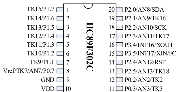
Figure 1-4 SOP20/TSSOP20 引脚配置图
