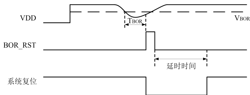
Figure 6-1 BOR 示意图
