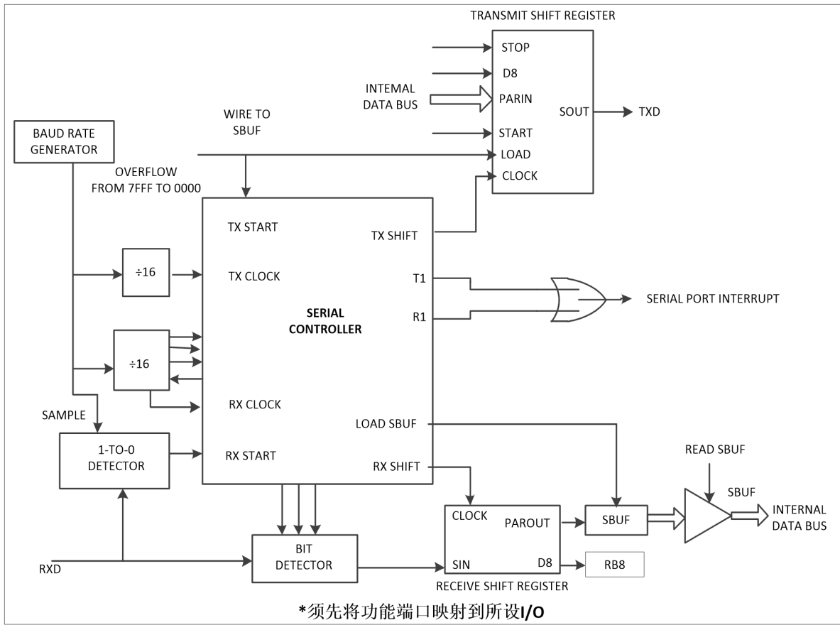
ure 13- 10 UART 模式 3 功能框图
