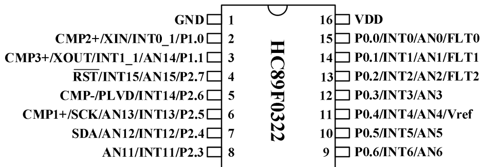
Figure 1-3 SOP16 引脚配置图
