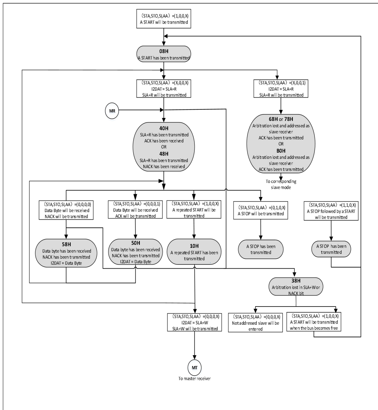
Figure 16- 10 主机接收模式流程与状态
