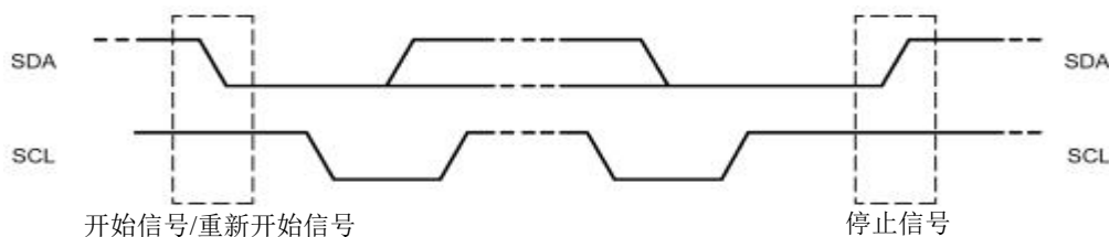
Figure 16-4 开始、重新开始、停止信号
