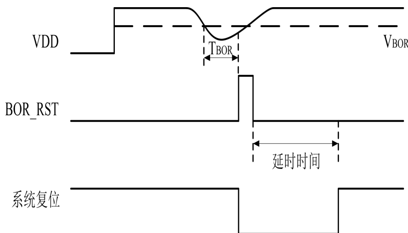
Figure 6-1 BOR 示意图
