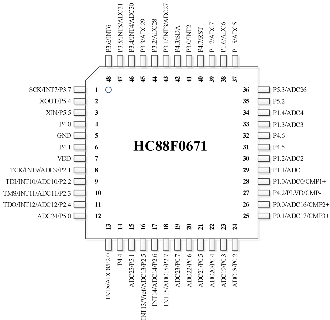
Figure 1-2 LQFP48 引脚配置图
