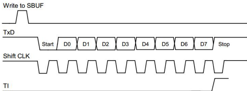
Figure 14-5 模式 1 数据发送时序框图
