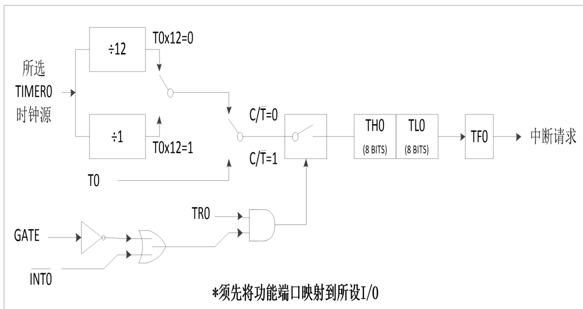
re 9-2 TIMER0 方式 1 功能框图
