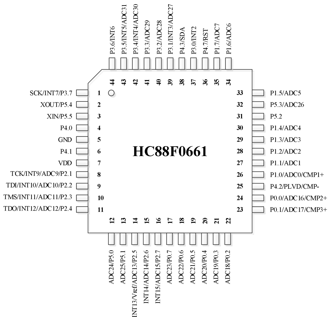
Figure 1-3 LQFP44 引脚配置图
