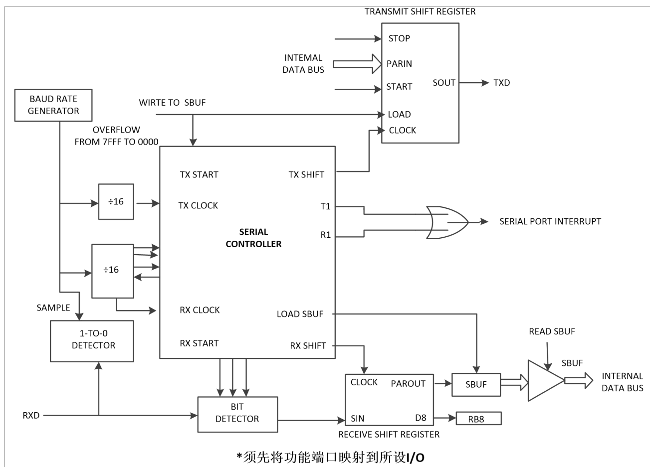
Figure 14-4 UART 模式 1 功能框图
