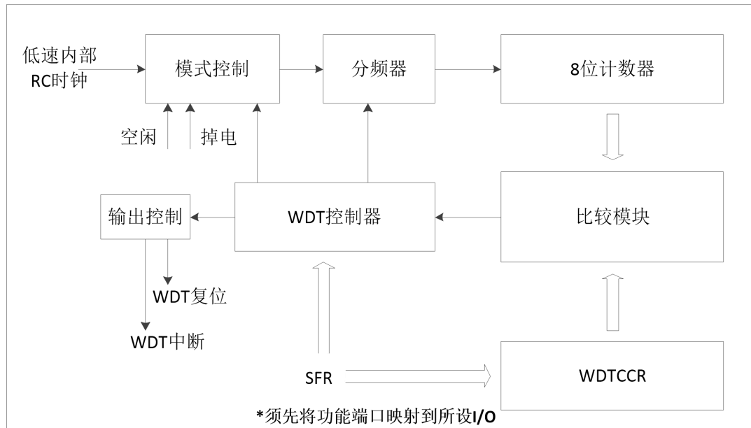
ure 13-1 WDT 功能框图
