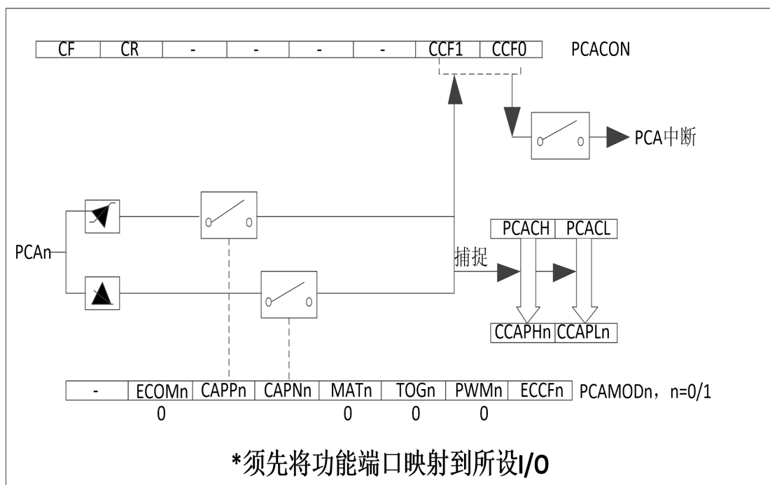
Figure 12-1 PCA 捕获模式图
