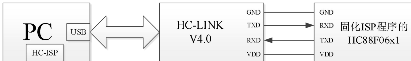
Figure 25- 1 ISP 串口烧录框图
