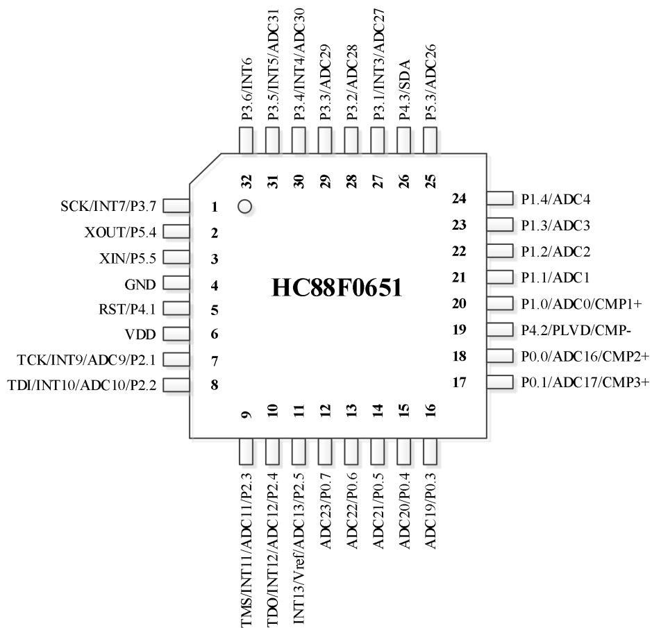
Figure 1-4 LQFP32 引脚配置图
