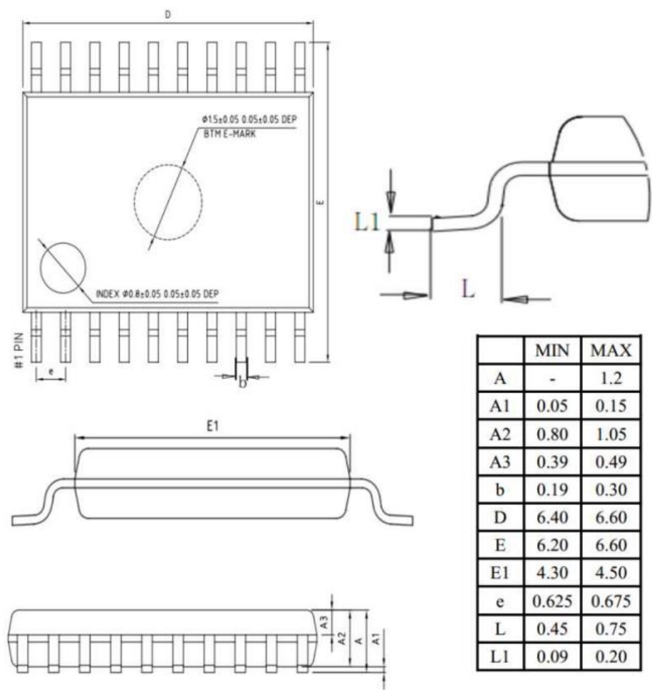
Figure 19-3 TSSOP20 封装尺寸
