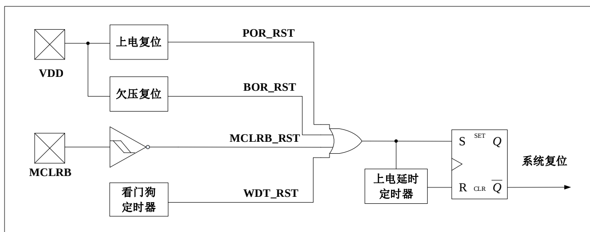
Figure 6-1 复位电路示意图
