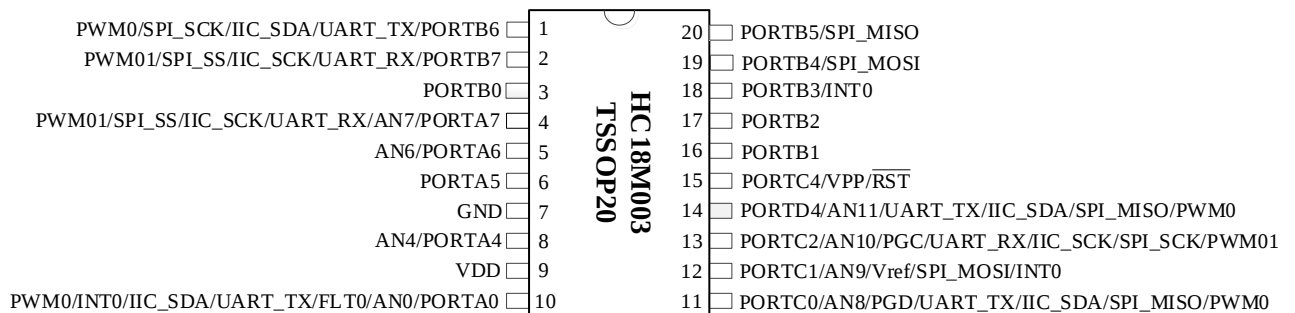
Figure 1-4 TSSOP20 引脚配置图
