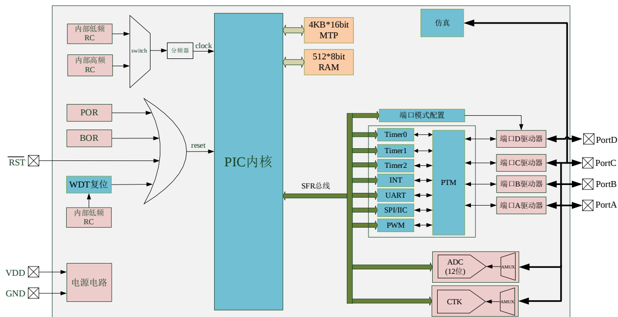
Figure 1-1 系统框图
