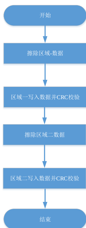
图 3-1 擦写操作
