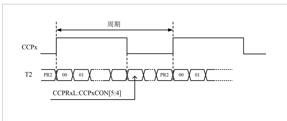
图8-8 PWM波形图
