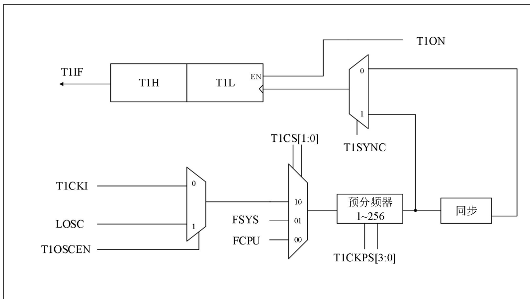
图8-3Timer1模块框图
