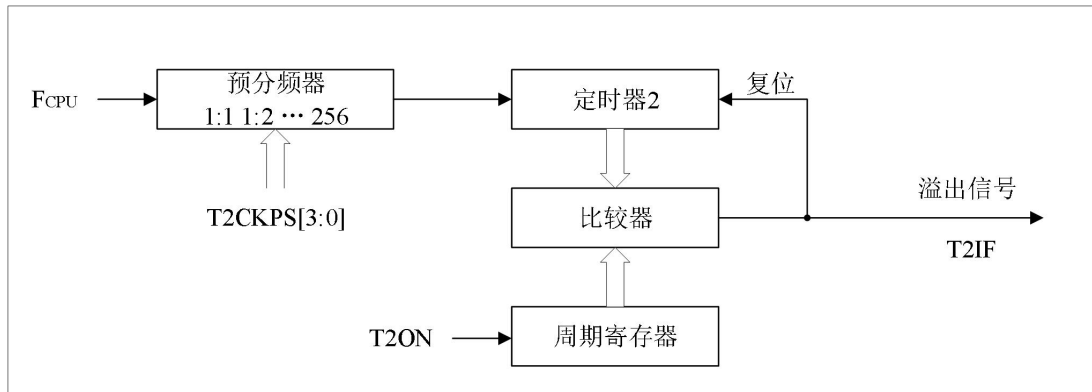
图8-4 Timer2模块框图
