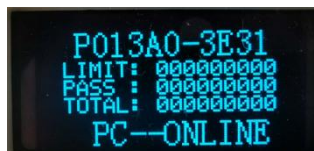
图 3.2-5 HC-PM18-V5 显示屏确认芯片型号及芯片特征码
