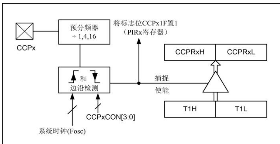
捕捉模式工作原理图：
