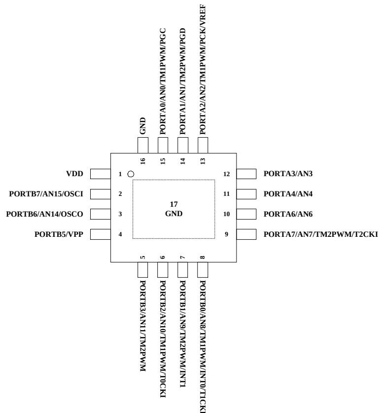
SQL5821B-QFN16 引脚配置图
