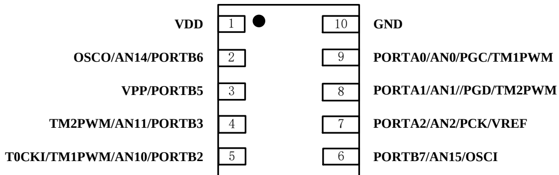
SQL5820B-MSOP10 引脚配置图
