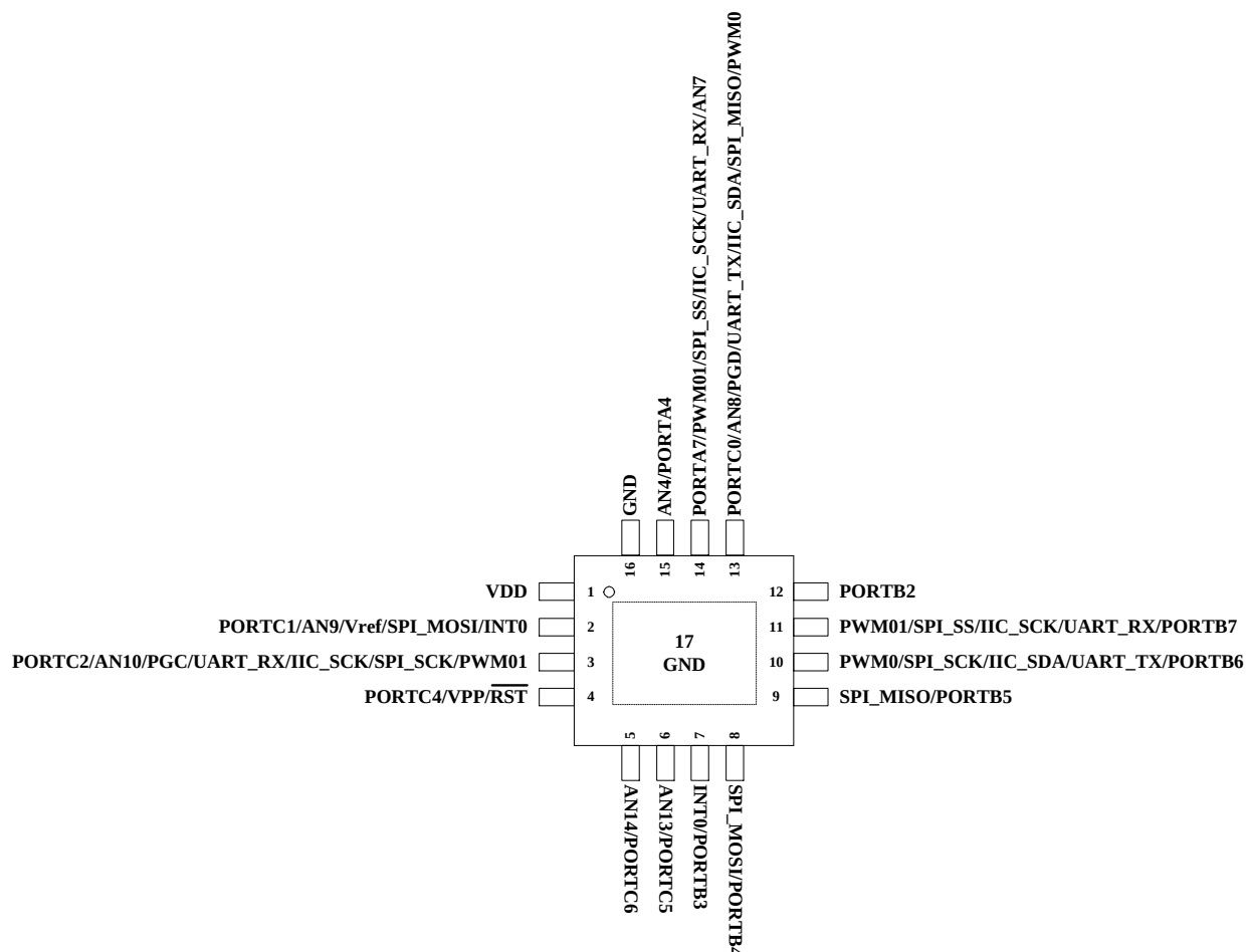
Figure 1-2 QFN16(3*3)引脚配置图
