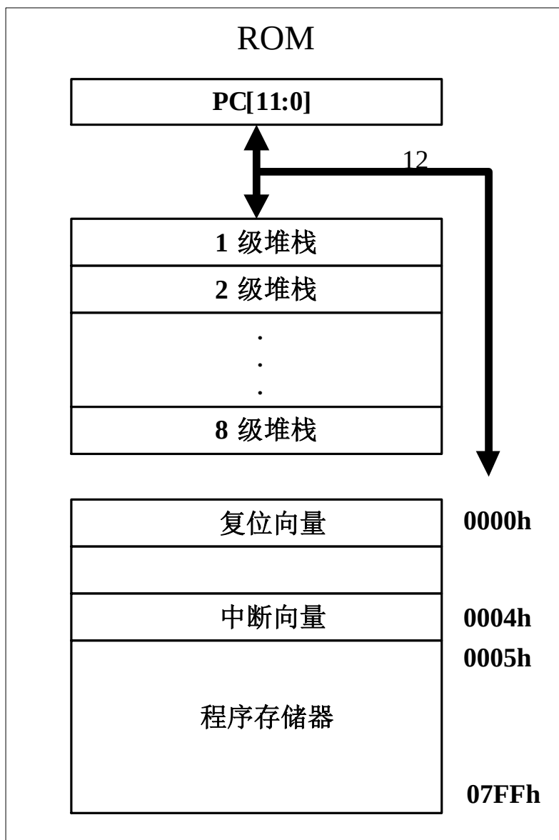
Figure 3-1 MTP 结构图
