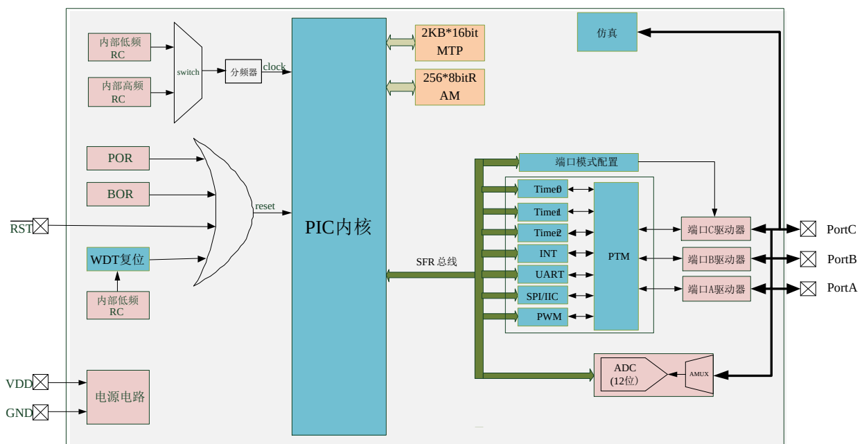
Figure 1-1 系统框图
