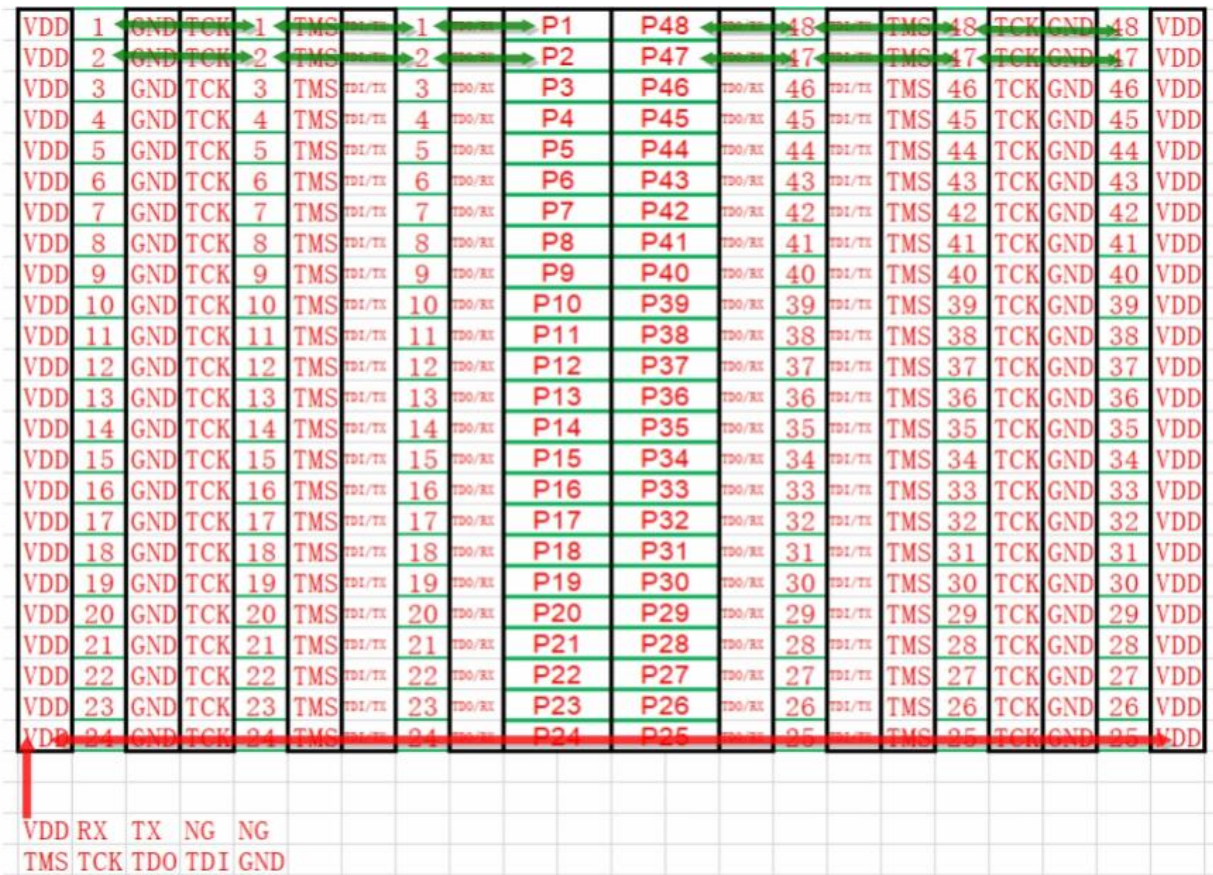
图 6-1 烧录转接板脚位示意图
